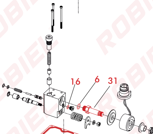
Válvula Reguladora Pressão Bomba C7/C9 Pressure Valve Cat C7/C9 HEUI High Pressure Pump 340.19.04
